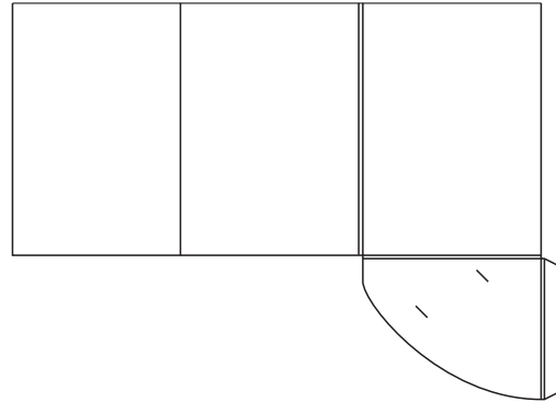
Stanzform O34: 215x305mm, 1 Klappe, 5mm Füllhöhe, Visitenkartenschlitze
