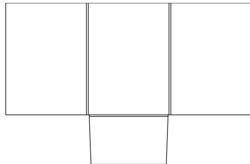
Stanzform O38: 220x305mm, 2 Klappen, 5mm Füllhöhe
