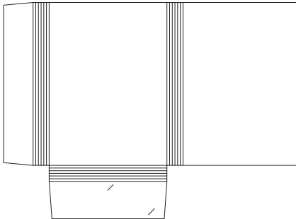
Stanzform 011: 220x305mm, 2 Klappen, Visitenkartenschlitze, 30mm Füllhöhe
