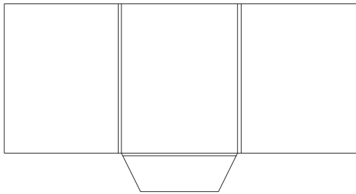
Stanzform O17: 220x283mm, 2 Klappen, 7mm Füllhöhe
