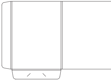
Stanzform O19: 220x305mm, 2 Klappen, Visitenkartenschlitze, 6mm Füllhöhe
