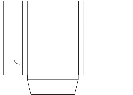
Stanzform O36: 215x310mm, 2 Klappen, 20mm Füllhöhe
