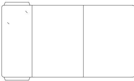
Stanzform 013: 220x310mm, 1 Klappe mit 2 Klebelaschen, Visitenkartenschlitze, 5mm Füllhöhe
