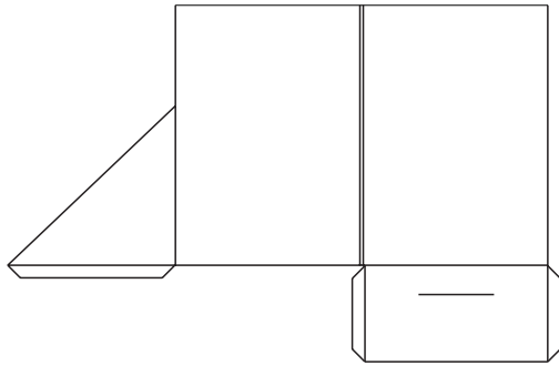
Stanzform O33: 220x310mm, 2 Klappen, Visitenkartenschlitze, 4mm Füllhöhe
