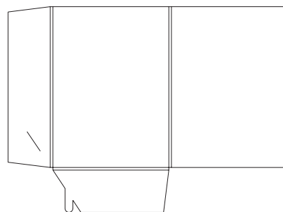
Stanzform 008: 220x305mm, 2 Klappen, 5mm Füllhöhe
