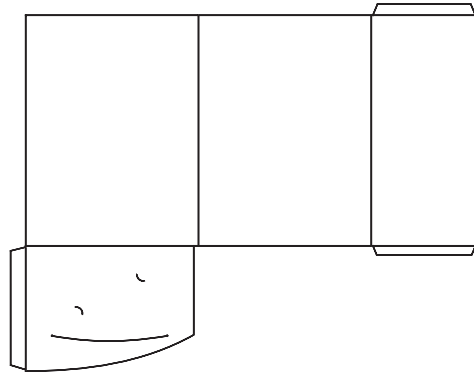
Stanzform O44: 219x305mm, 2 Klappen, Visitenkartenschlitze, CD-Schlitz
