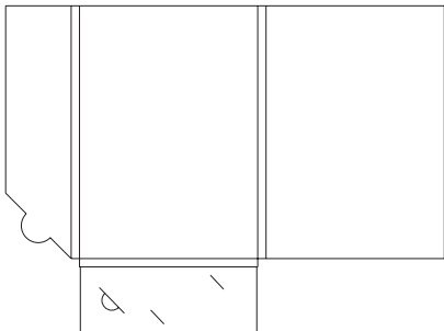
Stanzform O29: 215x305mm, 2 Klappen, Visitenkartenschlitze, 10mm Füllhöhe
