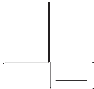
Stanzform O48: 220x310mm, 2 Klappen, 5mm Füllhöhe, CD-Schlitz
