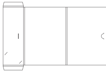
Stanzform 014: 212x300mm, 1 Klappe, 2 Klebelaschen, Visitenkartenschlitze, 6,5mm Füllhöhe
