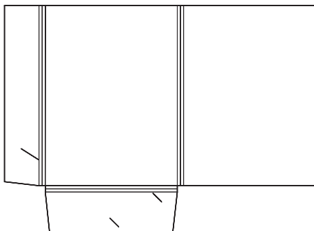
Stanzform O47: 230x310mm, 2 Klappen, 11mm Füllhöhe, Visitenkartenschlitze
