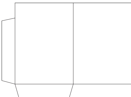
Stanzform O31: 220x305mm, 2 Klappen
