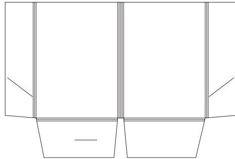
Stanzform O18: 218x310mm, 4 Klappen, 60mm Schlitz, 16mm Füllhöhe
