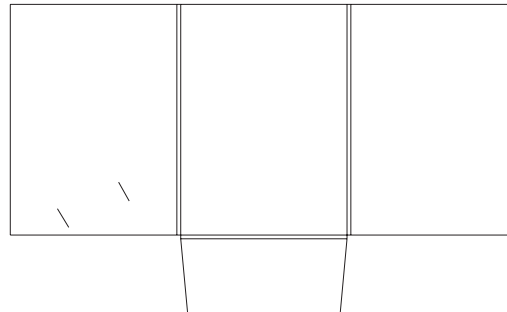
Stanzform O28: 220x305mm, 2 Klappen, Visitenkartenschlitze, 5mm Füllhöhe
