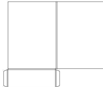
Stanzform O30: 220x307mm, 1 Tasche mit 2 Klebelaschen, 5mm Füllhöhe
