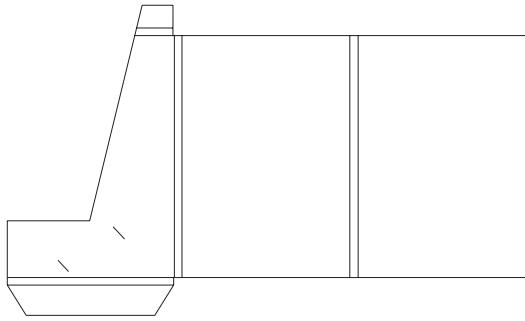
Stanzform O25: 222x320mm, 1 Klappe mit 2 Klebelaschen, Visitenkartenschlitze, 10mm Füllhöhe
