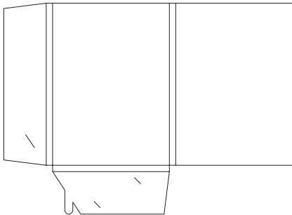
Stanzform O27: 220x305mm, 2 Klappen, Visitenkartenschlitze, 12mm Füllhöhe
