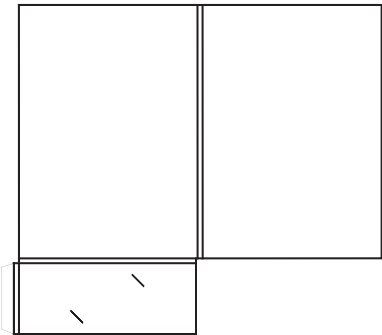
Stanzform O43: 215x305mm, 1 Klappe, Visitenkartenschlitze, 6mm Füllhöhe
