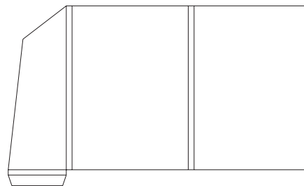
Stanzform 016: 220x310mm, 1 Klappen, 1 Klebelasche, 11mm Füllhöhe
