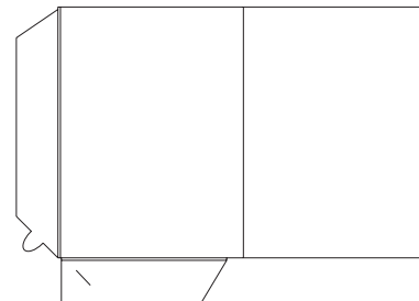
Stanzform 004: 220x302mm, 2 Klappen, 3mm Füllhöhe
