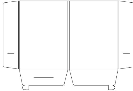
Stanzform O26: 220x308mm, 4 Klappen, 90mm Schlitz, 8mm Füllhöhe
