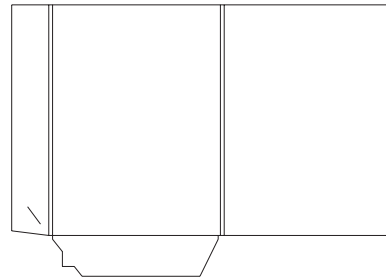
Stanzform O20: 222x305mm, 2 Klappen, 5mm Füllhöhe
