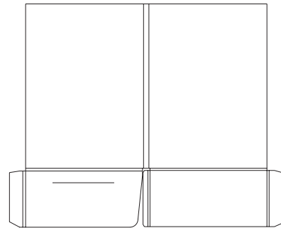
Stanzform O22: 220x307mm, 2 Taschen mit 2 Klebelaschen, 115mm Schlitze, 10mm Füllhöhe
