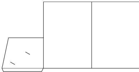
Stanzform O35: 220x305mm, 1 Klappe, Visitenkartenschlitze
