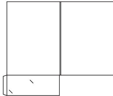
Stanzform O46: 220x305mm, 1 Klappe, Visitenkartenschlitze, 4mm Füllhöhe
