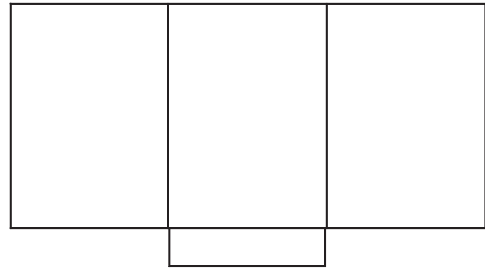
Stanzform O42: 210x297mm, 2 Klappen
